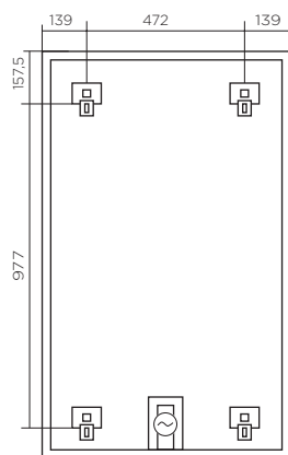
RETRO IN VERTICALE 750 x 1230 mm ⊙ Allacciamento rete
