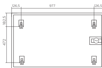
RETRO IN ORIZZONTALE 1230 x 750 mm ⊙ Allacciamento rete
